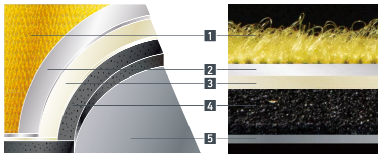
AGTitan210® 五層構造
